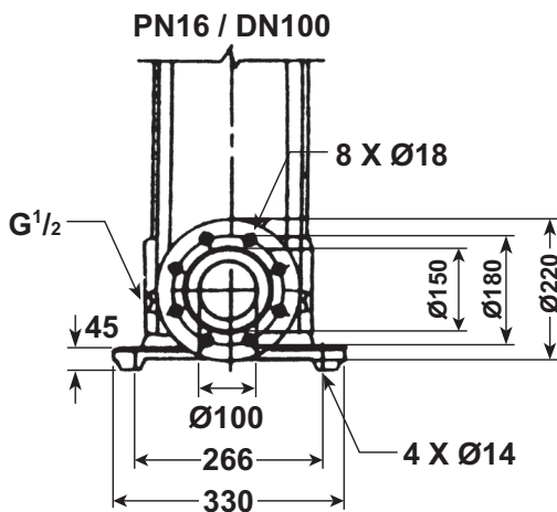
VM65 – PN16
