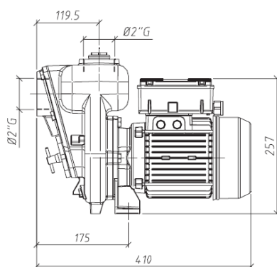
EB92 (1Φ)
